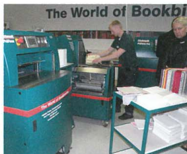
In einer Linie: Einhängen, Falzeinbrennen und Pressen mit Prä-Endfertigungsmaschinen von Schmedt.
